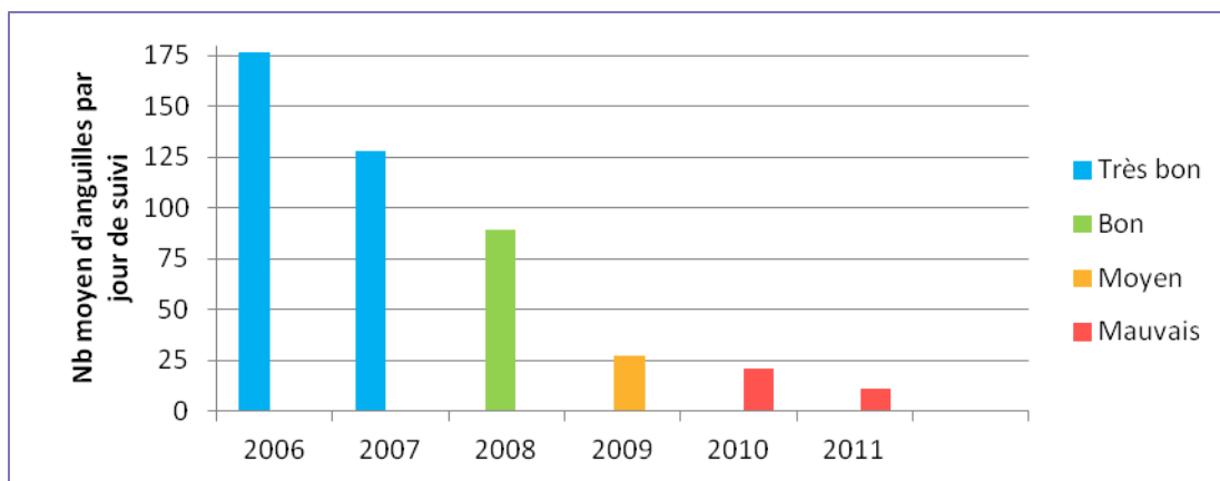
Figure 6 : Moyenne annuelle de l'indice de migration sur l'ensemble des passes fluviales de Vendée. Les seuils de référence sont calculés sur l'ensemble des données disponibles (2006-2011). Données FVPPMA 2012.
