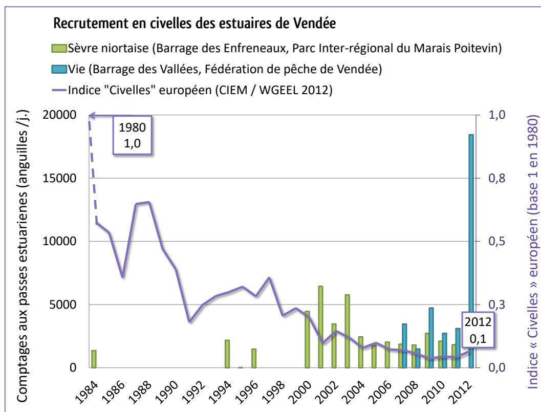
Figure 5 : Indices de migration (effectifs moyens par jour de suivi sur la période avril à juillet) observés sur les passes estuariennes de Vendée (données : FDPPMA de Vendée 2012) et de la Sèvre niortaise (données : Parc Interrégional du Marais Poitevin 2011). Source : ROUL 2012 (LOGRAMI – FVPPMA85).
