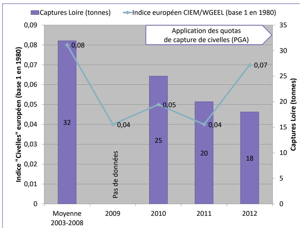
Figure 4 : Comparaison de l'indice « civelles » européen, hors Mer du Nord (base 1 = 1960-1979, source CIEM/WGEEL 2012) et les captures de civelles déclarées par la pêche professionnelle de l'estuaire de la Loire (Source : DDEA Loire-Atlantique 2008, Onema 2010, MAAPRAT/MEEDDTL 2011, MEDDE 2012), sur les saisons 2003-2004 à 2011-2012.
