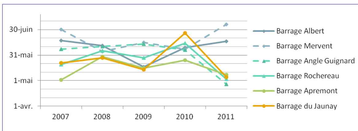
Figure 7 : Evolution de la date médiane des franchissements des passes fluviales de Vendée. Données FVPPMA 2012.
