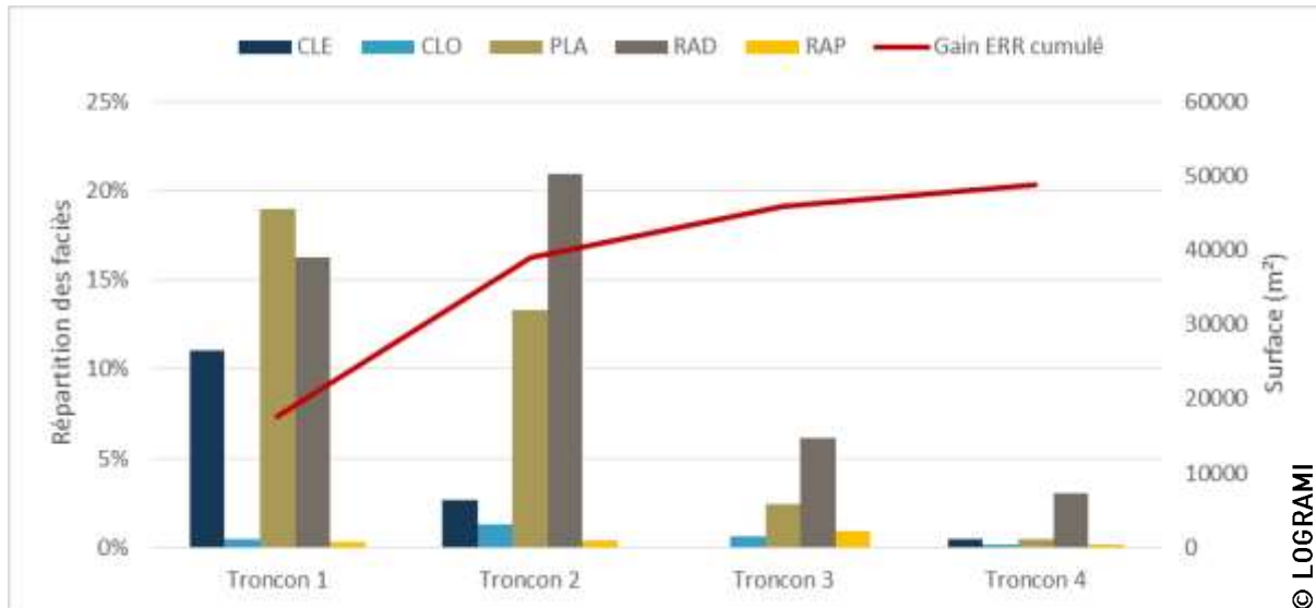
Figure 31 : Répartition longitudinale des faciès par tronçon et gain cumulé en ERR de la Couze d'Ardes
